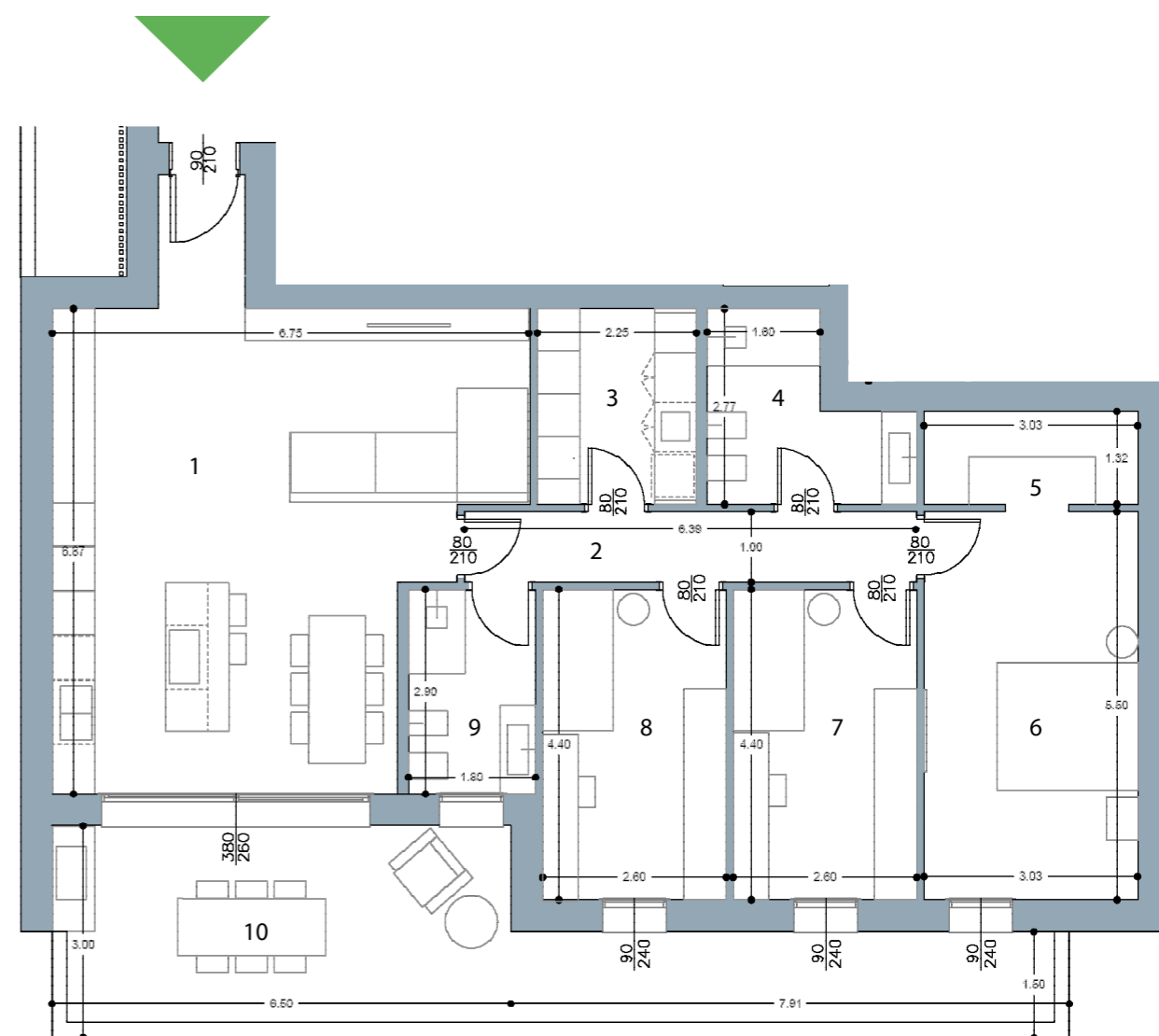
PLANIMETRIA SCALA 1:100
