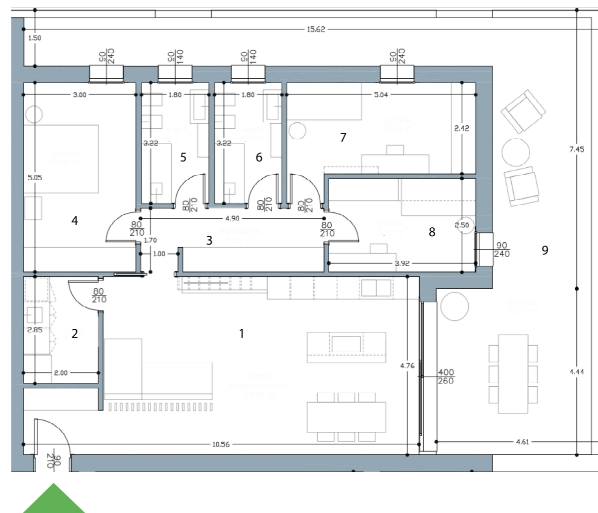
PLANIMETRIA SCALA 1:100
