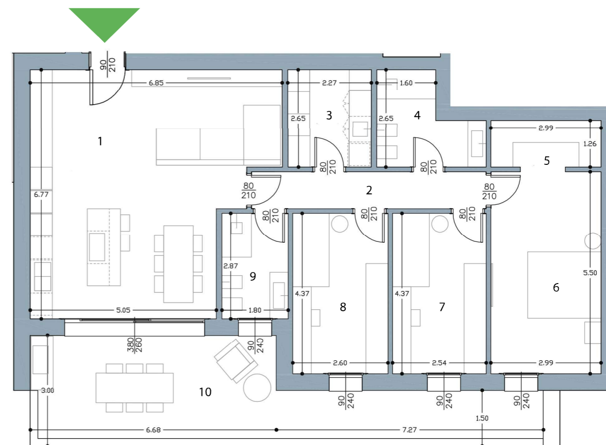
PLANIMETRIA SCALA 1:100
