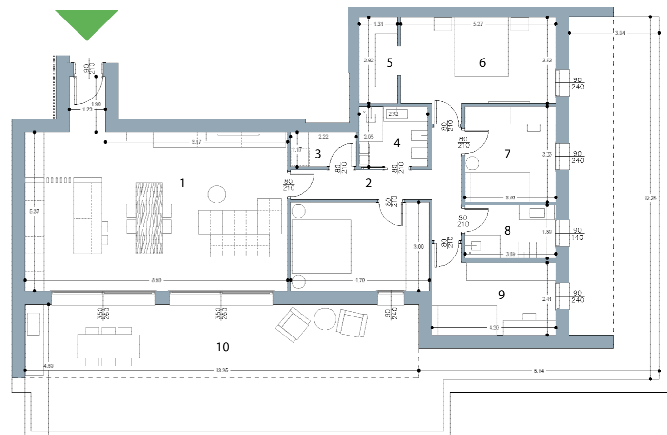
PLANIMETRIA SCALA 1:100
