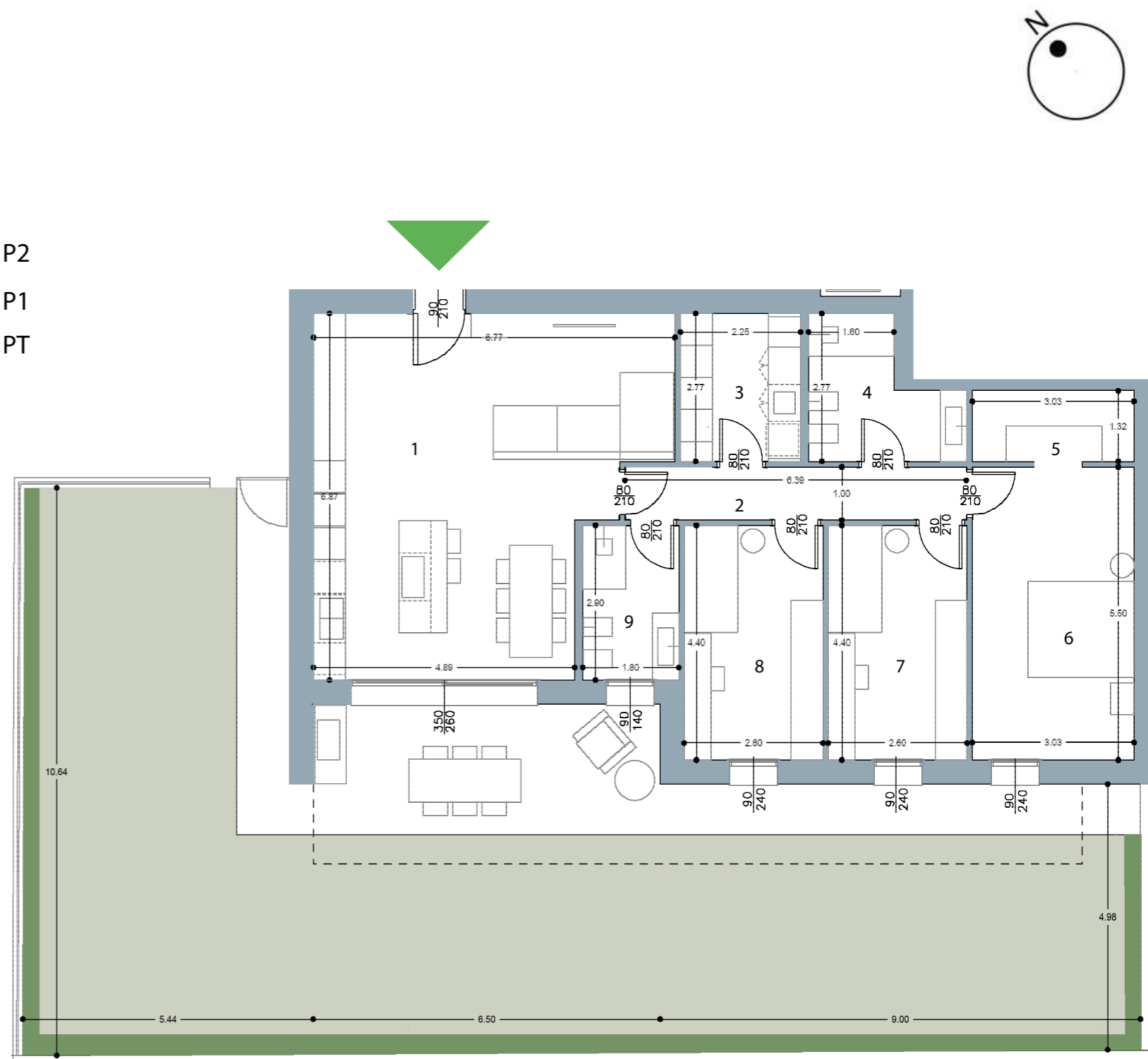
PLANIMETRIA SCALA 1:100
