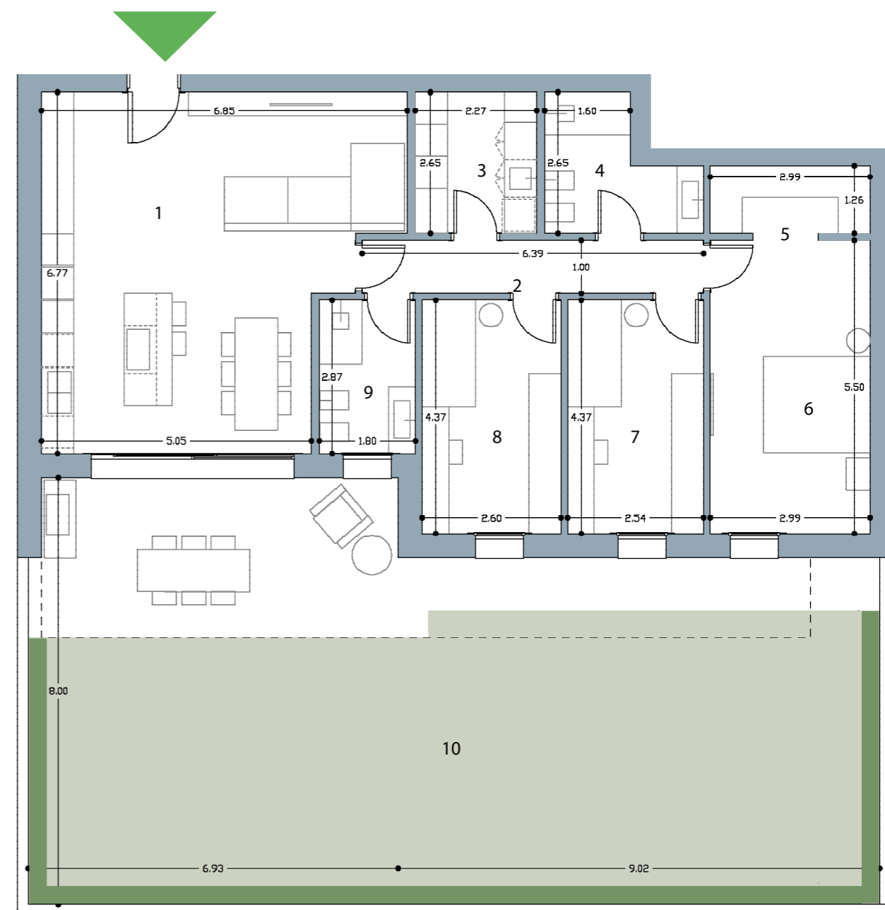
PLANIMETRIA SCALA 1:100
