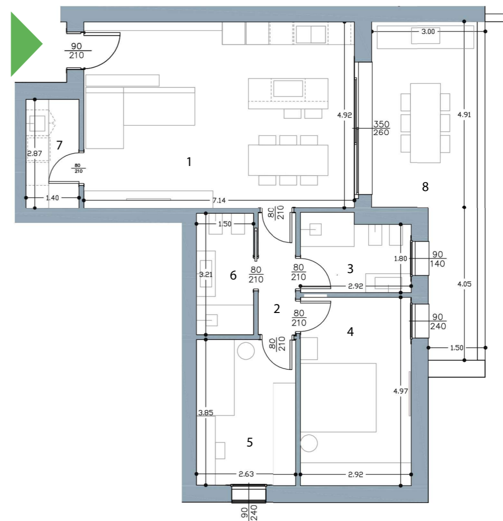
PLANIMETRIA SCALA 1:100
