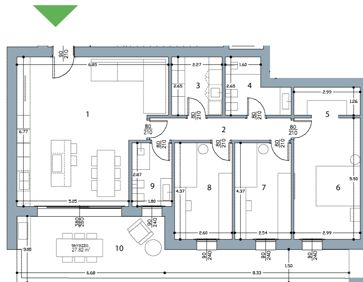
PLANIMETRIA SCALA 1:100
